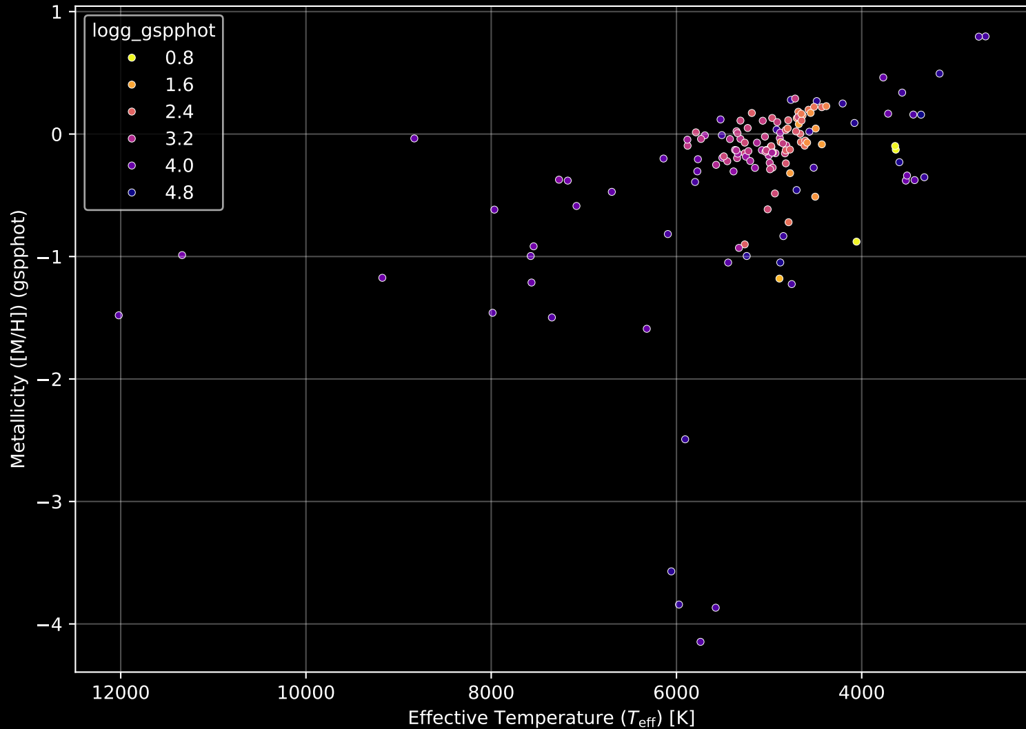
APOGEE DR17 Field: [TAUL1495_btx] Stellar Population Parameters (n= 143)
